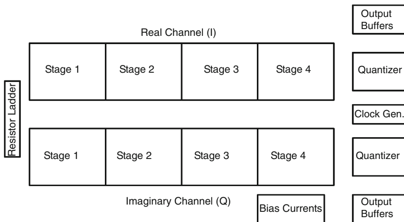
Fig. 5.14 Modulator floor-plan
