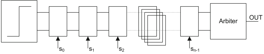
Fig. 1.9 Arbiter PUF
